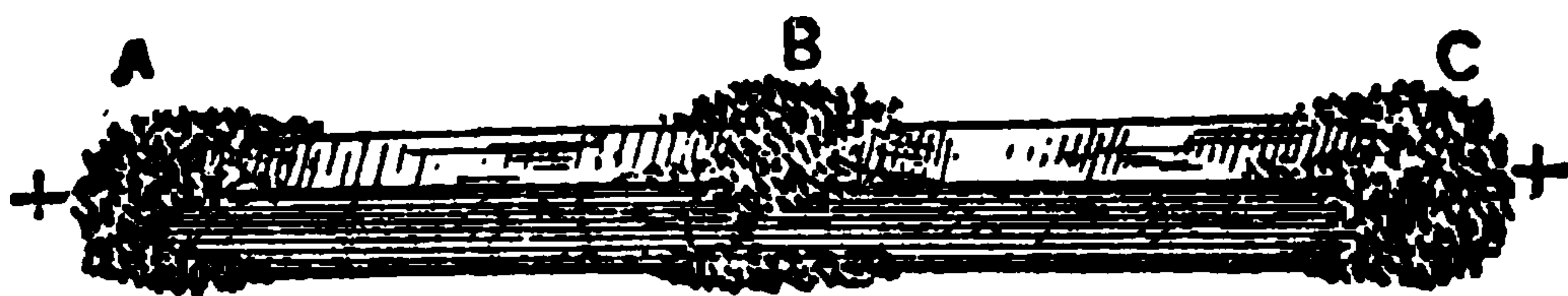
FIG. 45.—ANOMALOUS MAGNET.
